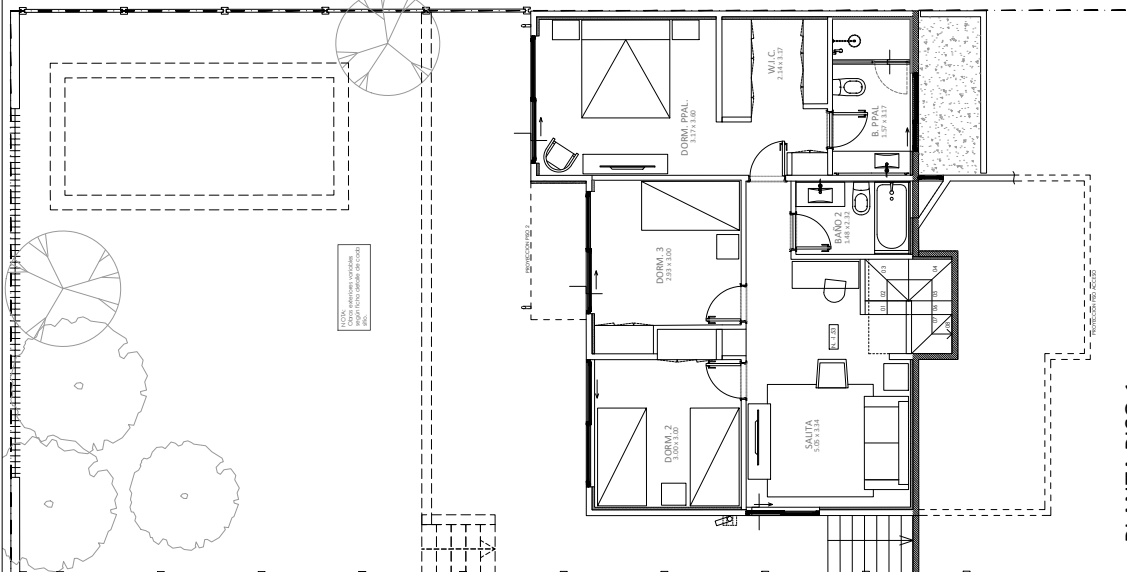
PLANTA PISO 1 ESC 1/100
